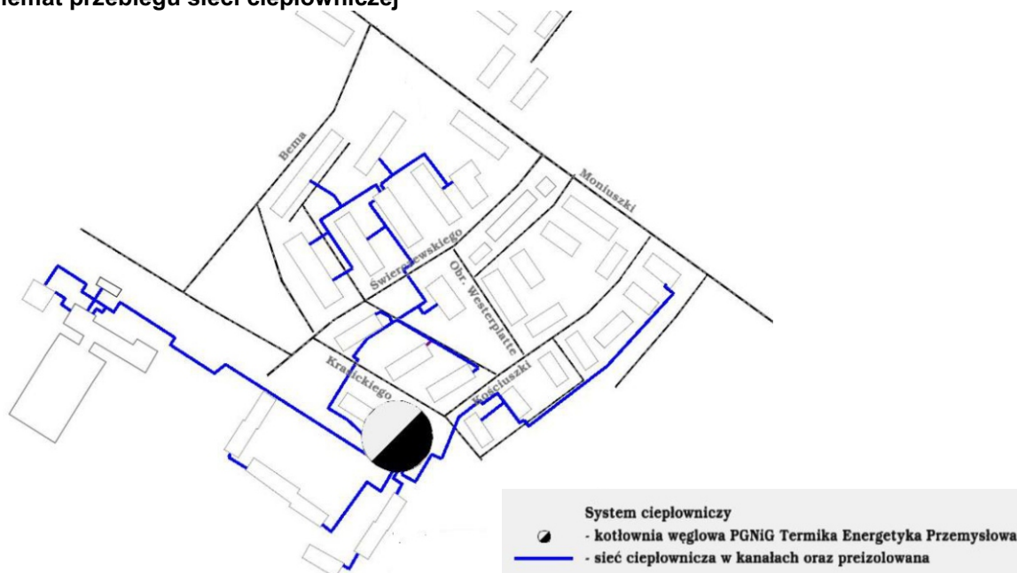
Rysunek 4-1 Schemat przebiegu sieci ciepłowniczej
