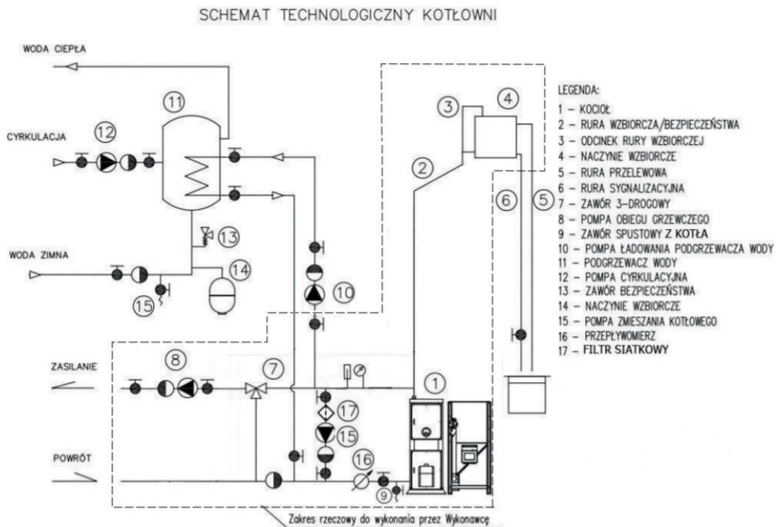
Rys. 2. Schemat kotłowni – układ otwarty
